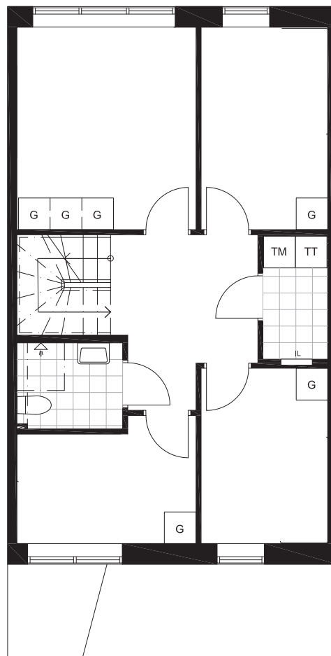
Ovanvåning
