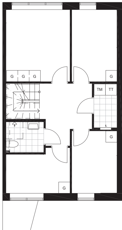
Ovanvåning
